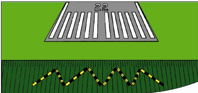
Bild 7. Markeringar på slutningar i omedelbar anslutning till tröskeln
