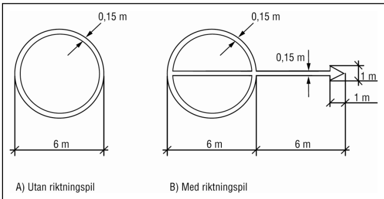
Bild 11. Markering av VOR-kontrollplats
