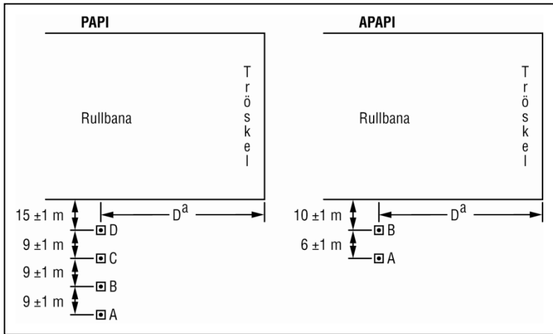
Bild 13. PAPI/APAPI-placering
