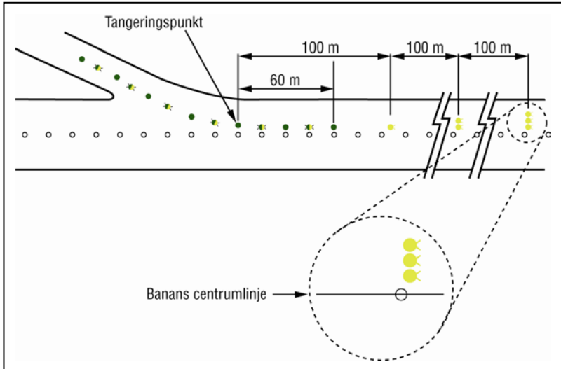
Bild 19. Varselljus för snabbavfartstaxibana
