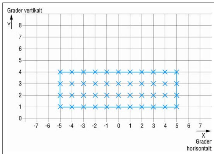
Bild 18. Rutnätspunkter för beräkning av medelljusstyrka hos centrumlinjeljus i taxibana och stoppljus.
