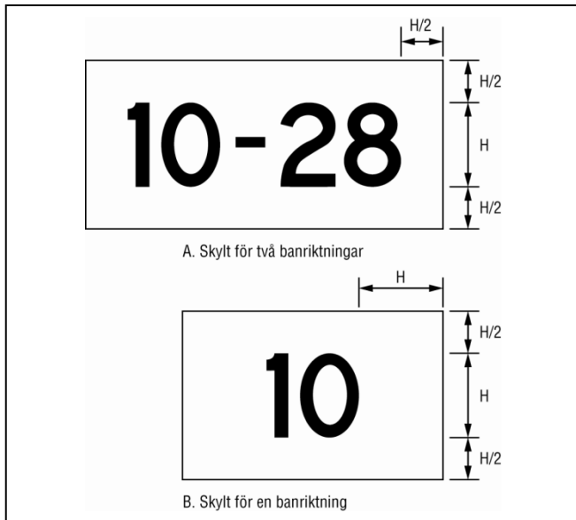
Bild 27. Skyltbredd
