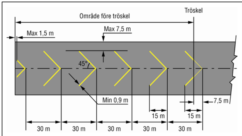
Bild 30. Vinkelmarkeringar
