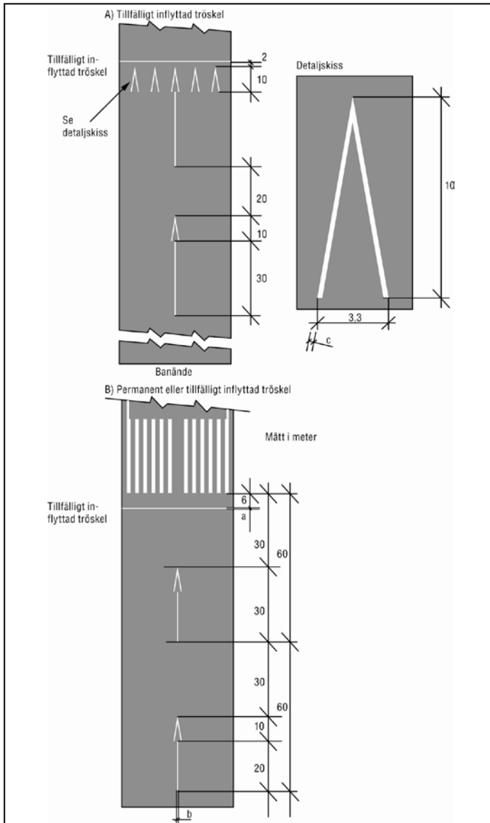
Bild 5. Inflyttade tröskel- markeringar
