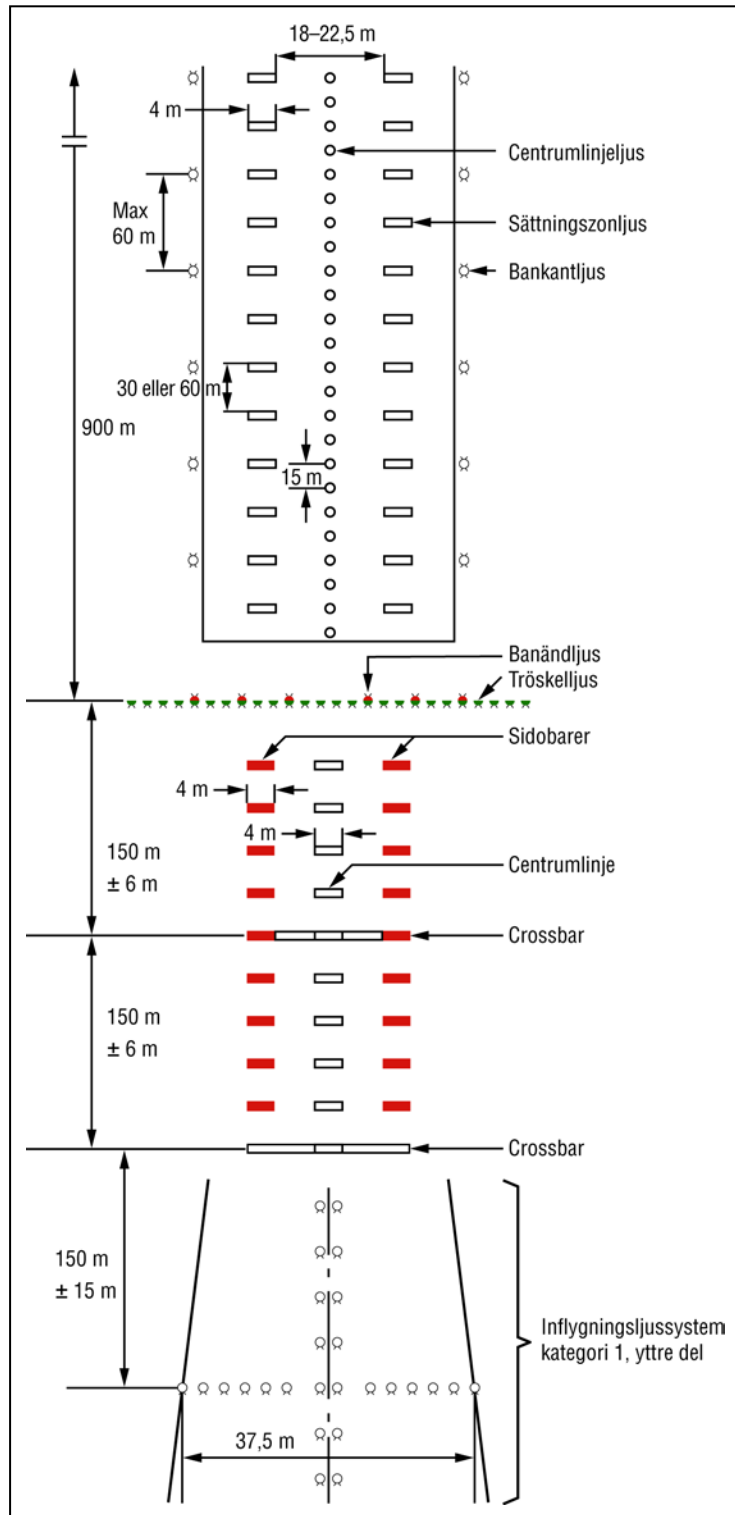
Bild 3. Inflygningsljussystem kategori II och III, inre delen samt anslutande del av banljus
