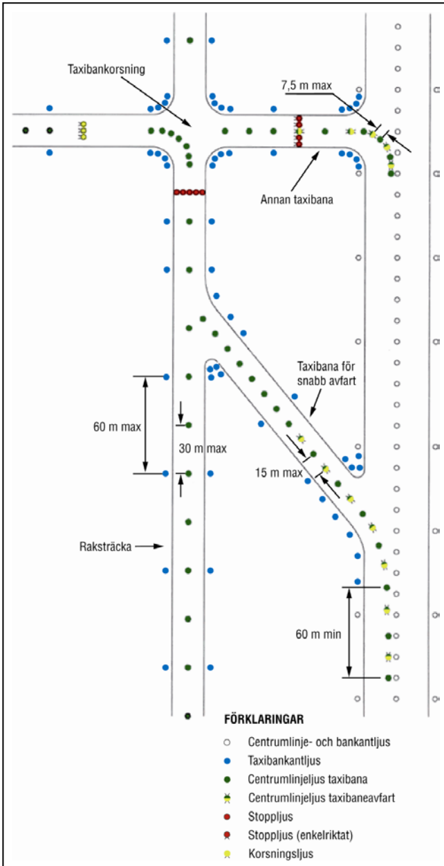
Bild 21. Taxibanljus
