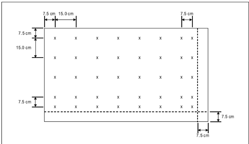
Bild 26. Gridpunkter för mätning av luminansmedelvärde.
